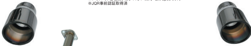
■VMG/VM4 Levorg 2.0/1.6 GT VMG/VM4 スポーツエキゾーストキット ¥205,200 (本体¥190,000) ※メインパイプφ60.5 - 50.8×2, 総重量:17.2kg, ※アウトレット左右出し(90-110φ 楕円×2), 3pcsセット, ※JQR事前認証取得済
