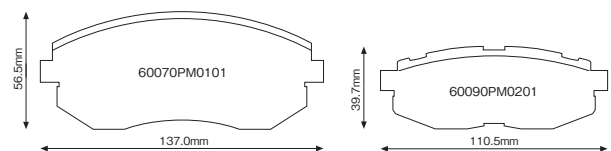
BM/BR 2.5GT, GRF/GVF A-Line ※Brembo非装着 系
